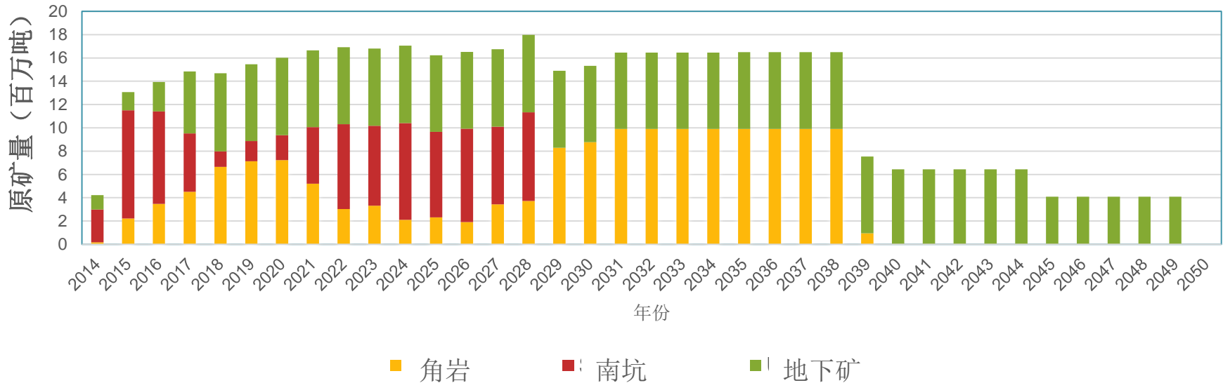
二期露天及地下采矿计划
